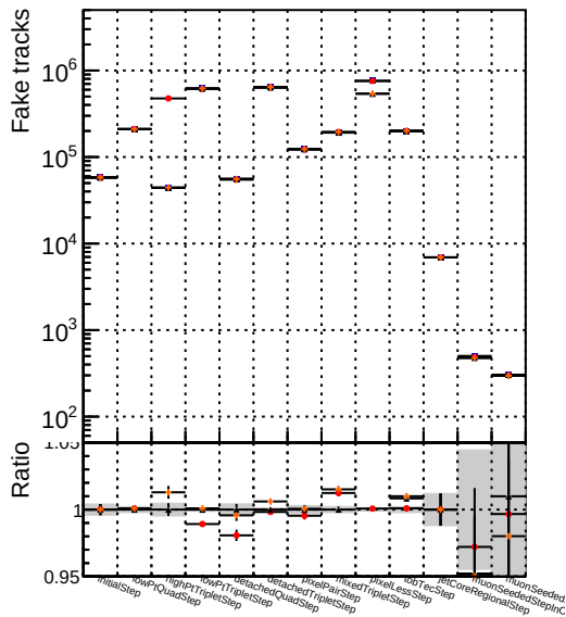
—●— DQM_mkFit TTbase —●— DQM_mkFit TT_retrainOldFiles125_v2_prelimWP_5iter —●— DQM_mkFit TT_baseline_6iter —●— DQM_mkFit TT_RetrainV2_WP1_6iter
