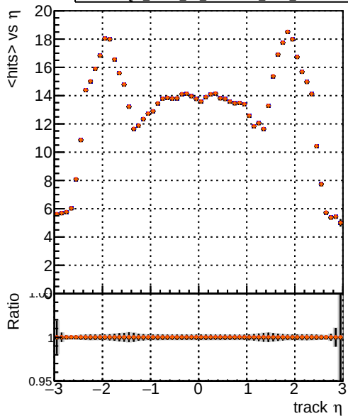
mean hit DQM_mkFit_TTbase DQM_mkFit_TT_retrainOldFiles125_v2_prelimWP_5iter DQM_mkFit_TT_baseline_6iter DQM_mkFit_TT_RetrainV2_WP1_6iter
