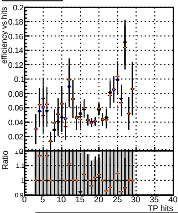
Efficiency vs hit Legend: DQM_mkFit_TTbase DQM_mkFit_TT_retrainOldFiles125_v2_prelimWP_5iter DQM_mkFit_TT_baseline_6iter DQM_mkFit_TT_RetrainV2_WP1_6iter
