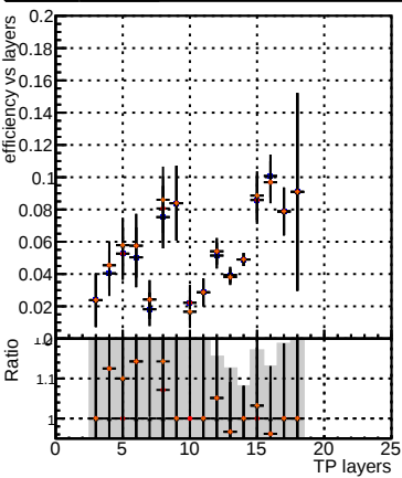
Efficiency vs hit Legend: DQM_mkFit_TTbase DQM_mkFit_TT_retrainOldFiles125_v2_prelimWP_5iter DQM_mkFit_TT_baseline_6iter DQM_mkFit_TT_RetrainV2_WP1_6iter
