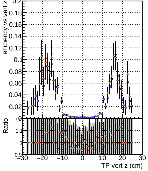
Efficiency vs vert z — DQM_mkFit TTbase — DQM_mkFit TT_retrainOldFiles125_v2_prelimWP_5iter — DQM_mkFit TT_baseline_6iter — DQM_mkFit TT_RetrainV2_WP1_6iter
