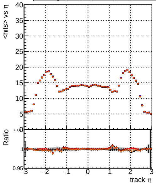
— DQM_mkFit_TTbase — DQM_mkFit_TT_retrainOldFiles125_v2_prelimWP_5iter — DQM_mkFit_TT_baseline_6iter — DQM_mkFit_TT_RetrainV2_WP1_6iter mean hits
