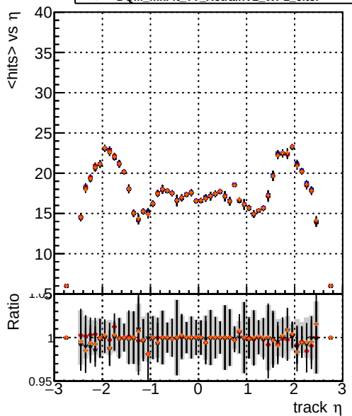
mean hits DQM_mkFit_TTbase DQM_mkFit_TT_retrainOldFiles125_v2_prelimWP_5iter DQM_mkFit_TT_baseline_6iter DQM_mkFit_TT_RetrainV2_WP1_6iter
