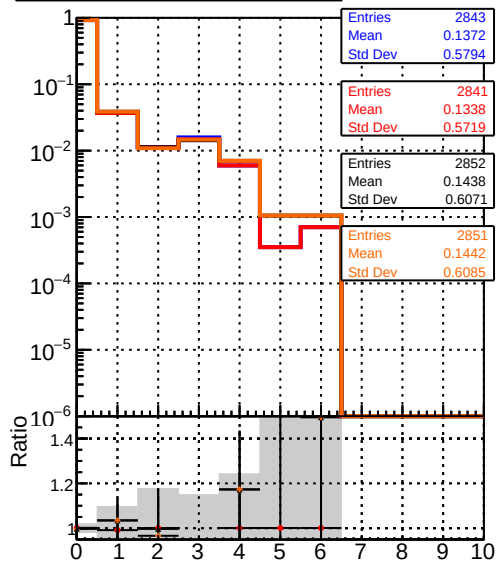
mean hits DQM_mkFit_TTbase DQM_mkFit_TT_retrainOldFiles125_v2_prelimWP_5iter DQM_mkFit_TT_baseline_6iter DQM_mkFit_TT_RetrainV2_WP1_6iter
