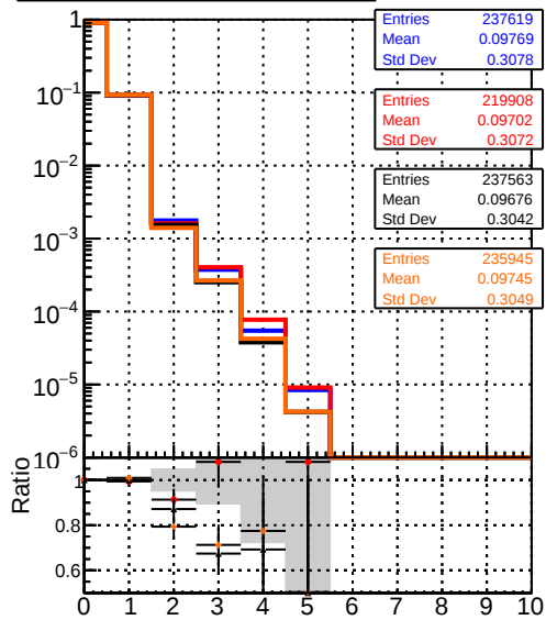
mean hit DQM_mkFit_TTbase DQM_mkFit_TT_retrainOldFiles125_v2_prelimWP_5iter DQM_mkFit_TT_baseline_6iter DQM_mkFit_TT_RetrainV2_WP1_6iter
