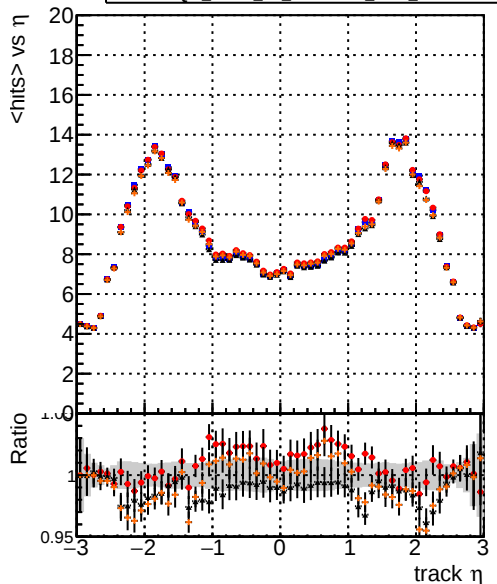
— DQM_mkFit_TTbase — DQM_mkFit_TT_retrainOldFiles125_v2_prelimWP_5iter — DQM_mkFit_TT_baseline_6iter — DQM_mkFit_TT_RetrainV2_WP1_6iter mean hit
