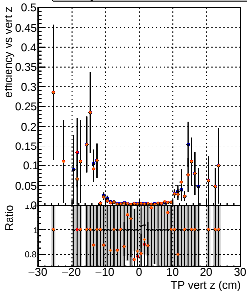
Efficiency vs. TP vert z (cm) Legend: - \bullet DQM_mkFit_TTbase - \circ DQM_mkFit_TT_retrainOldFiles125_v2_prelimWP_5iter - \star DQM_mkFit_TT_baseline_6iter - \times DQM_mkFit_TT_RetrainV2_WP1_6iter
