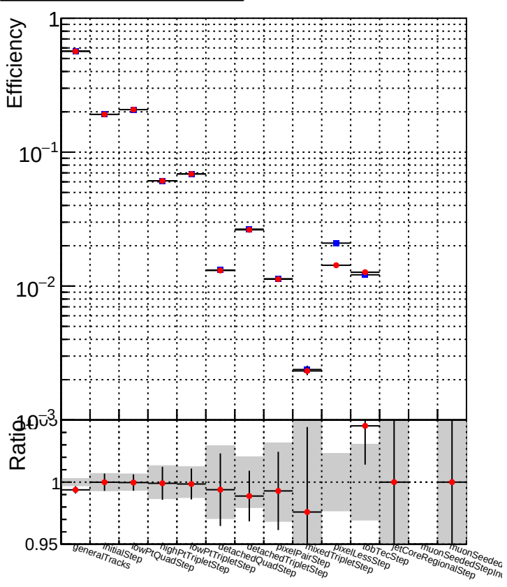
DQM_mkFit_baseline_lowPT DQM_mkFit_baseline6iter_lowPT
