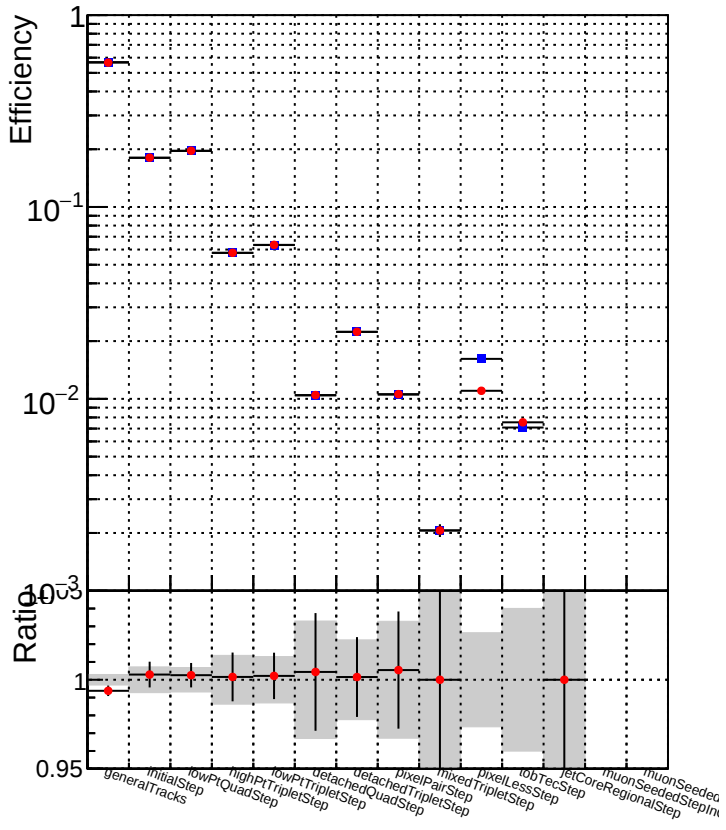
DQM_mkFit_baseline_lowPT DQM_mkFit_baseline6iter_lowPT
