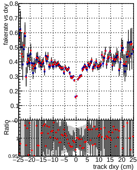
—•— DQM_mkFit_baseline_lowPT —•— DQM_mkFit_baseline6iter_lowPT
