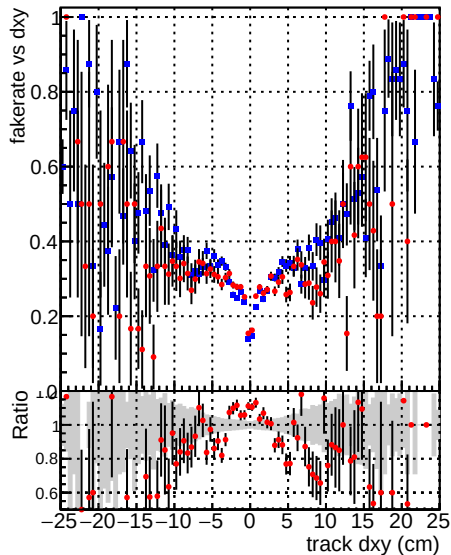
—◆— DQM_mkFit_baseline_lowPT —●— DQM_mkFit_baseline6iter_lowPT
