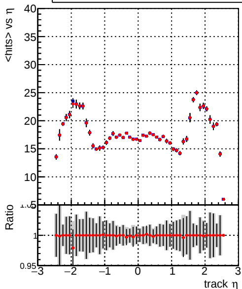
DQM_mkFit_baseline_lowPT mean hits DQM_mkFit_baseline6iter_lowPT
