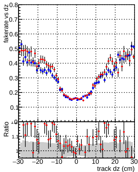
—◆— DQM mkFit baseline_lowPT —●— DQM mkFit baseline6iter_lowPT
