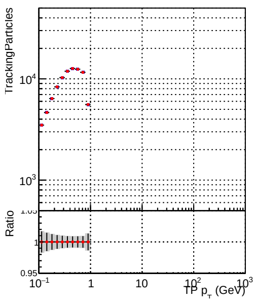
—•— DQM_mkFit_baseline_lowPT —•— DQM_mkFit_baseline6iter_lowPT
