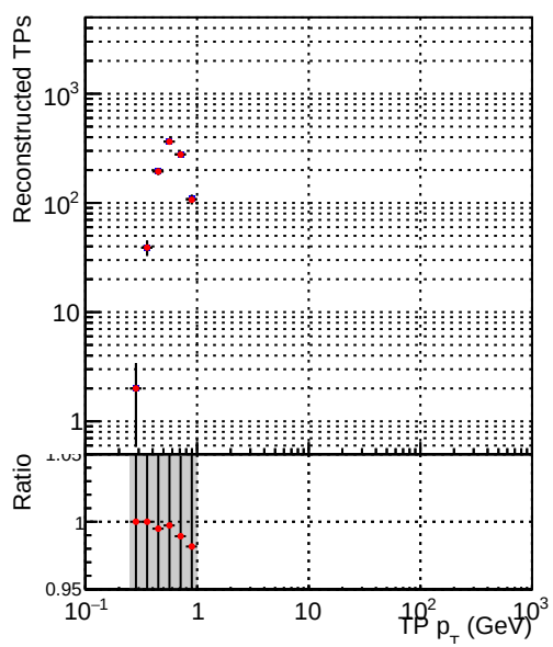
—•— DQM_mkFit_baseline_lowPT —•— DQM_mkFit_baseline6iter_lowPT
