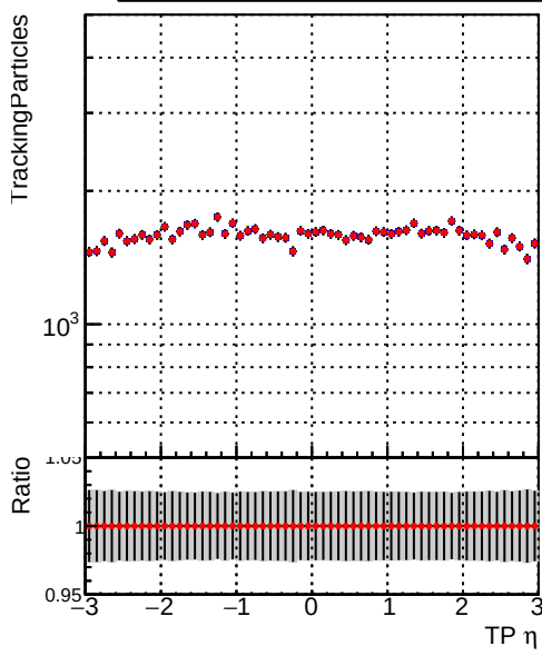
—•— DQM_mkFit_baseline_lowPT —•— DQM_mkFit_baseline6iter_lowPT
