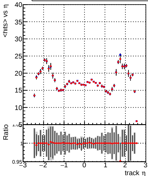
— DQM_mkFit_baseline_lowPT — DQM_mkFit_baseline6iter_lowPT
