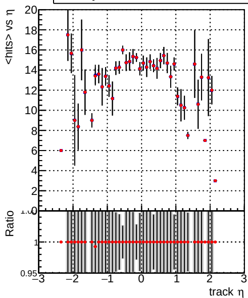
— DQM_mkFit_baseline_lowPT — DQM_mkFit_baseline6iter_lowPT
