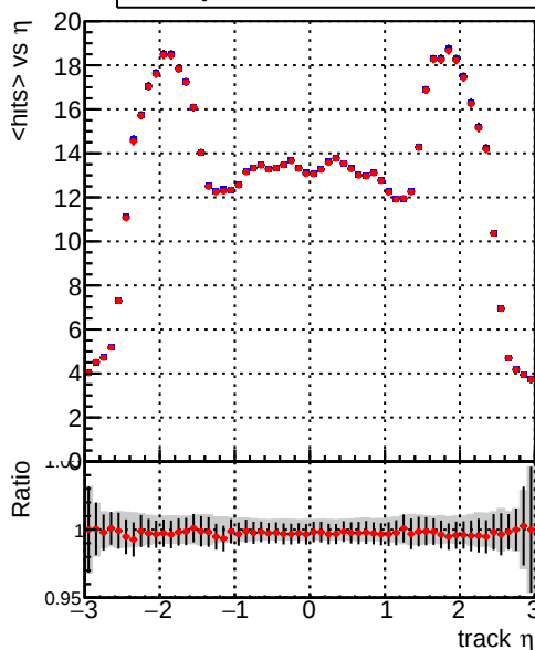
— DQM_mkFit_baseline_lowPT — DQM_mkFit_baseline6iter_lowPT
