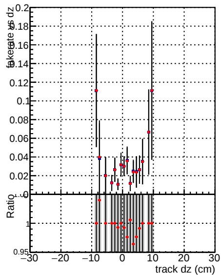
—•— DQM_mkFit_baseline_lowPT —•— DQM_mkFit_baseline6iter_lowPT
