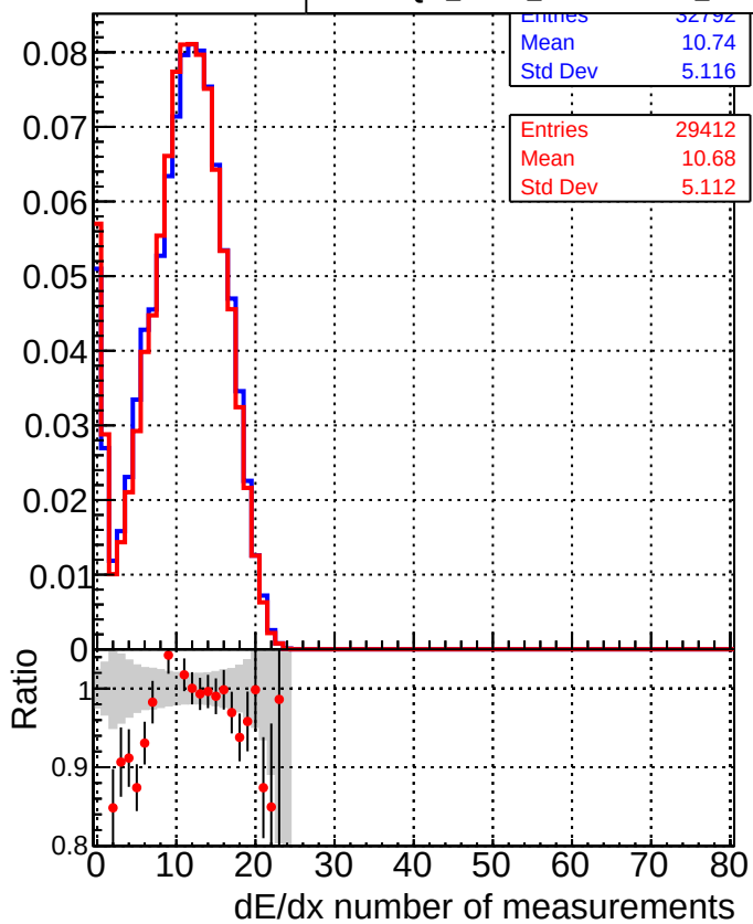
■ DQM_mkFit_baseline_lowPT ● DQM_mkFit_baseline6iter_lowPT
