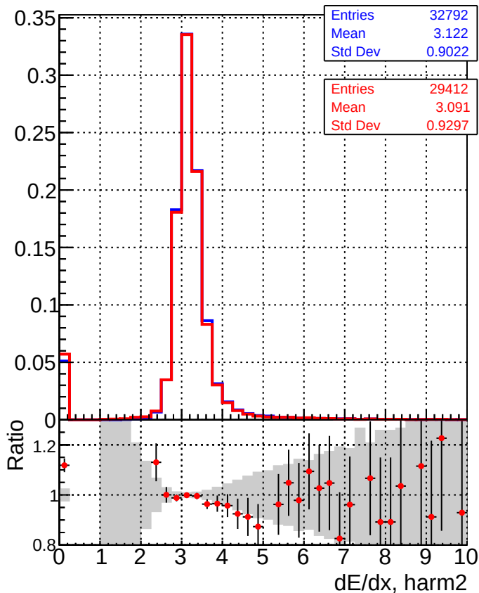
■ DQM_mkFit_baseline_lowPT ● DQM_mkFit_baseline6iter_lowPT
