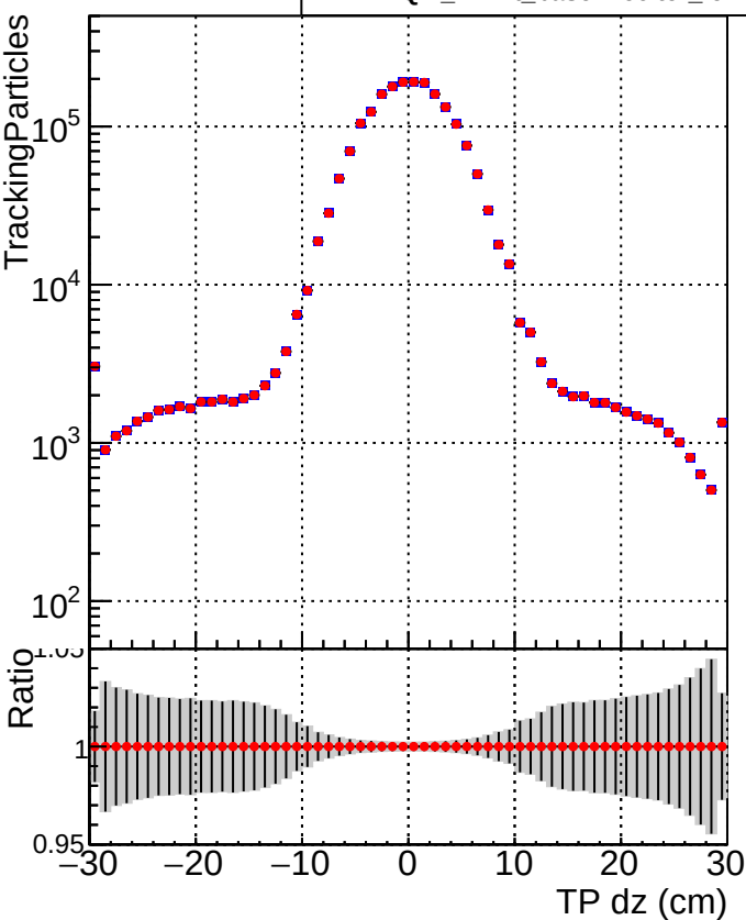
■ DQM_mkFit_baseline_lowPT ● DQM_mkFit_baseline6iter_lowPT
