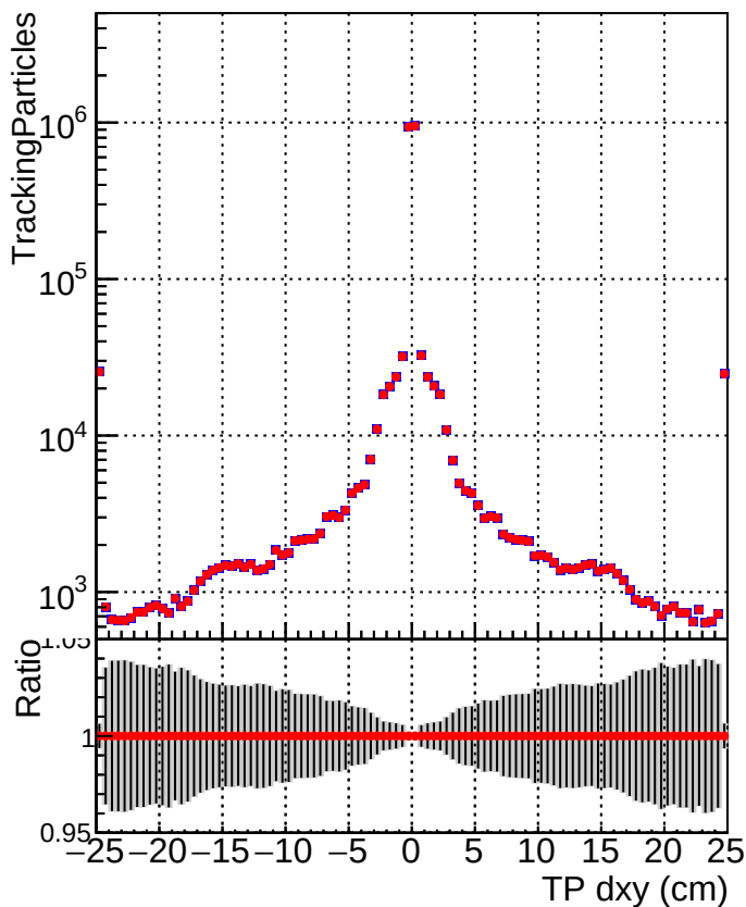
■ DQM_mkFit_baseline_lowPT ● DQM_mkFit_baseline6iter_lowPT
