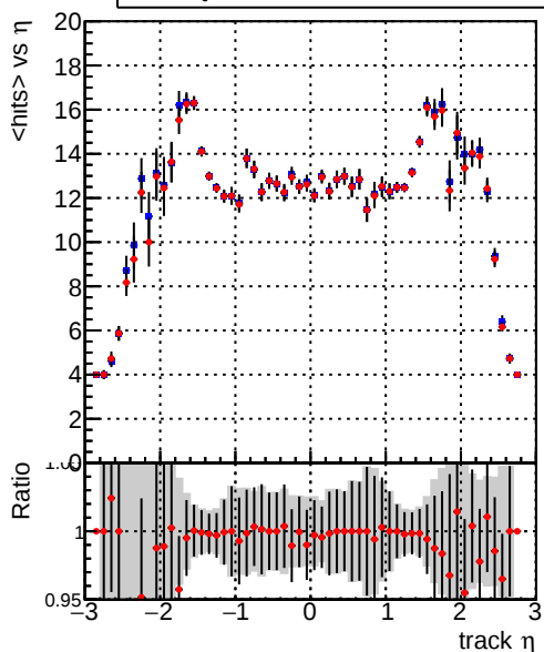
— DQM_mkFit_baseline_lowPT — DQM_mkFit_baseline6iter_lowPT
