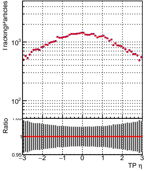
■ DQM_CKF_TTbase ■ DQM_mkFit_TTbase
