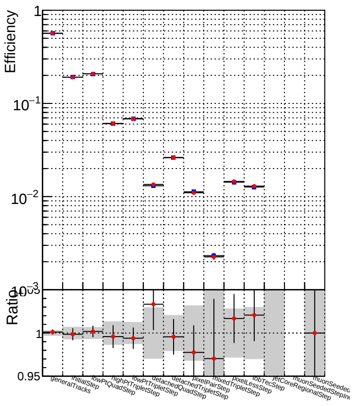
DQM_mkFit_TT_baseline_6iter DQM_mkFit_TT_RetrainV2_WP1_6iter
