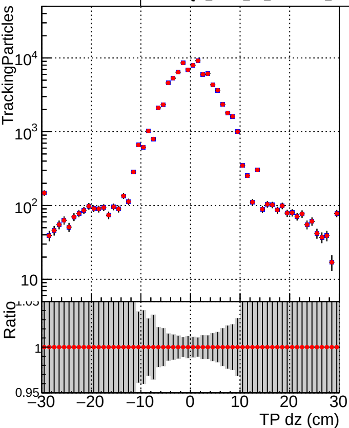
■ DQM_mkFit_TT_baseline_6iter ● DQM_mkFit_TT_RetrainV2_WP1_6iter
