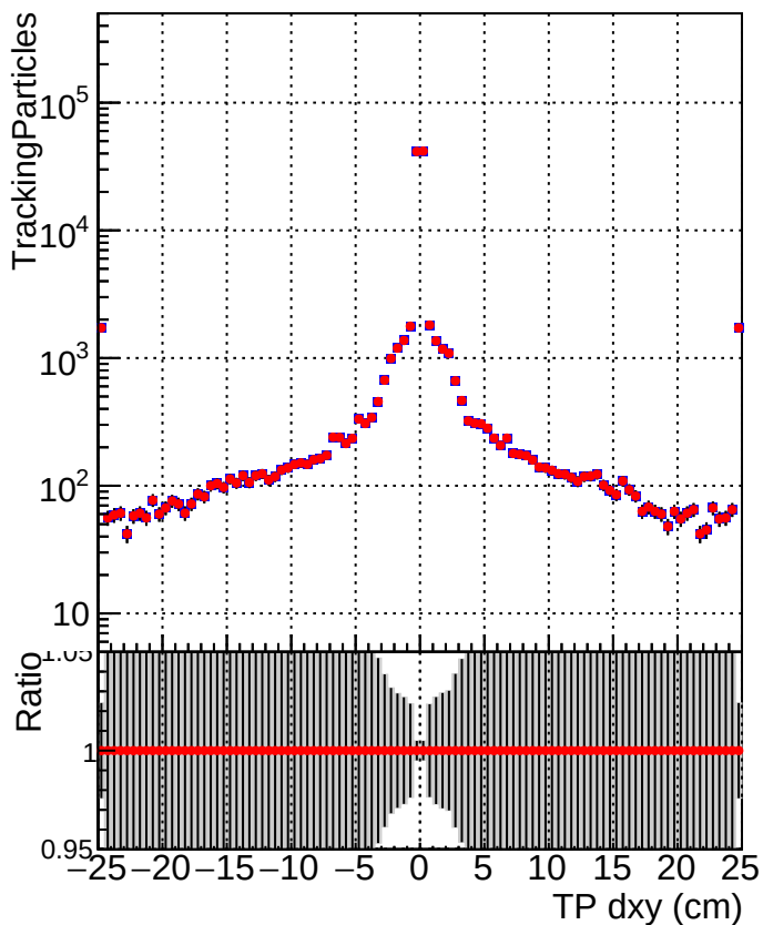
■ DQM_mkFit_TT_baseline_6iter ● DQM_mkFit_TT_RetrainV2_WP1_6iter
