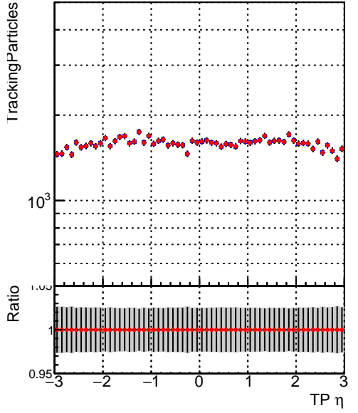
■ DQM_mkFit_TT_baseline_6iter ● DQM_mkFit_TT_RetrainV2_WP1_6iter
