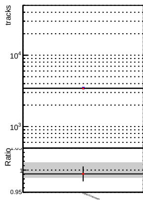
N of reco track vs. \chi^2 —●— DQM mkFit TT_baseline_6iter —●— DQM mkFit TT_RetrainV2_WP1_6iter
