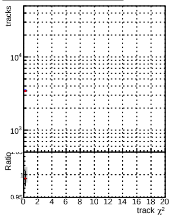
N of reco track vs. \chi^2 —●— DQM mkFit TT_baseline_6iter —●— DQM mkFit TT_RetrainV2_WP1_6iter
