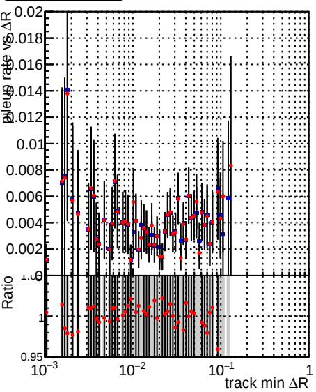
—•— DQM_mkFit_TT_baseline_6iter —•— DQM_mkFit_TT_RetrainV2_WP1_6iter
