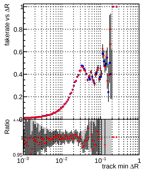
—•— DQM_mkFit_TT_baseline_6iter —•— DQM_mkFit_TT_RetrainV2_WP1_6iter
