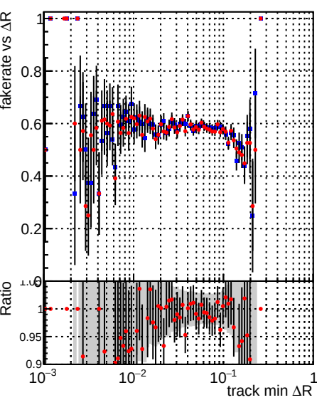
—•— DQM_mkFit_TT_baseline_6iter —•— DQM_mkFit_TT_RetrainV2_WP1_6iter
