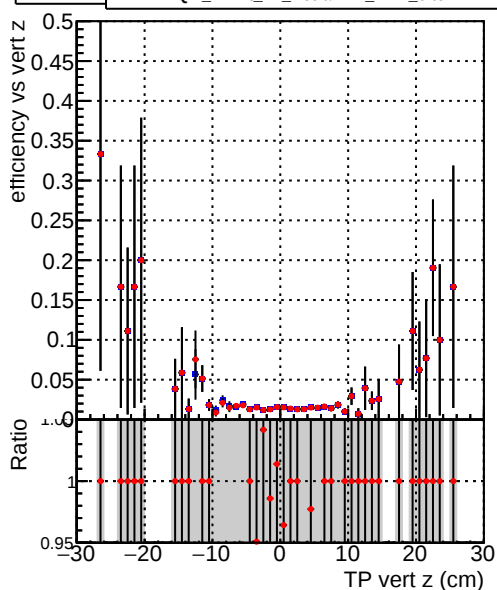
Efficiency vs. TP vert z (cm) — DQM_mkFit_TT_baseline_6iter — DQM_mkFit_TT_RetrainV2_WP1_6iter
