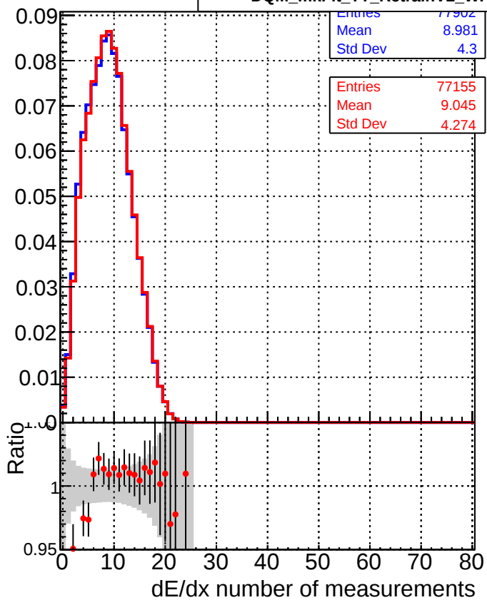
■ DQM_mkFit_TT_baseline_6iter ● DQM_mkFit_TT_RetrainV2_WP1_6iter
