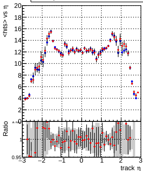
— DQM_mkFit_TT_baseline_6iter — DQM_mkFit_TT_RetrainV2_WP1_6iter mean hits
