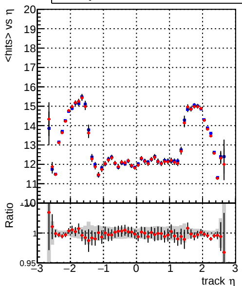
mean hits — DQM_mkFit_TT_baseline_6iter — DQM_mkFit_TT_RetrainV2_WP1_6iter
