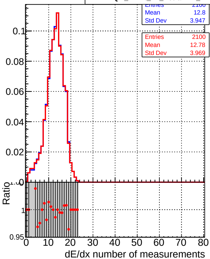
■ DQM_mkFit_TT_baseline_6iter ● DQM_mkFit_TT_RetrainV2_WP1_6iter
