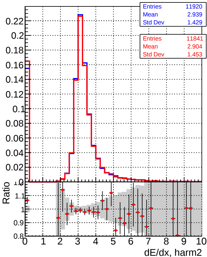
■ DQM_mkFit_TT_baseline_6iter ● DQM_mkFit_TT_RetrainV2_WP1_6iter
