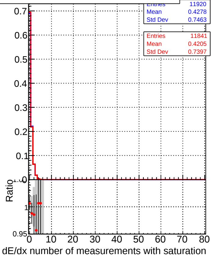
■ DQM_mkFit_TT_baseline_6iter ● DQM_mkFit_TT_RetrainV2_WP1_6iter
