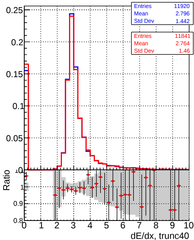
■ DQM_mkFit_TT_baseline_6iter ● DQM_mkFit_TT_RetrainV2_WP1_6iter
