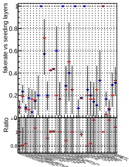
Fake rate vs. —♦— DQM mkFit TT baseline_6iter —★— DQM mkFit TT RetrainV2_WP1_6iter
