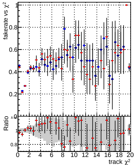
Fake rate vs. —♦— DQM mkFit TT baseline_6iter —★— DQM mkFit TT RetrainV2_WP1_6iter
