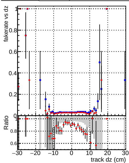
—●— DQM_mkFit_TT_baseline_6iter —●— DQM_mkFit_TT_RetrainV2_WP1_6iter
