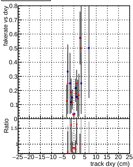
—●— DQM_mkFit_TT_baseline_6iter —●— DQM_mkFit_TT_RetrainV2_WP1_6iter
