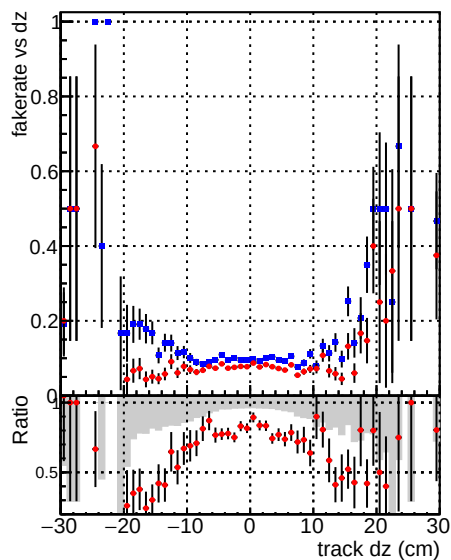
—●— DQM_mkFit_TT_baseline_6titer —●— DQM_mkFit_TT_RetrainV2_WP1_6titer
