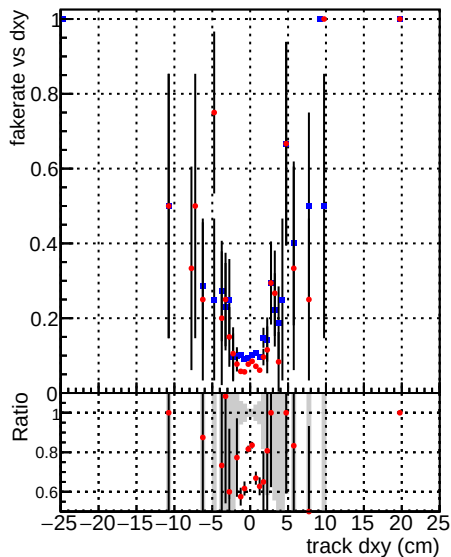
—●— DQM_mkFit_TT_baseline_6titer —●— DQM_mkFit_TT_RetrainV2_WP1_6titer
