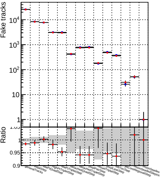
Number —●— DQM_mkFit_TT_RetrainV2_WP1_6iter
