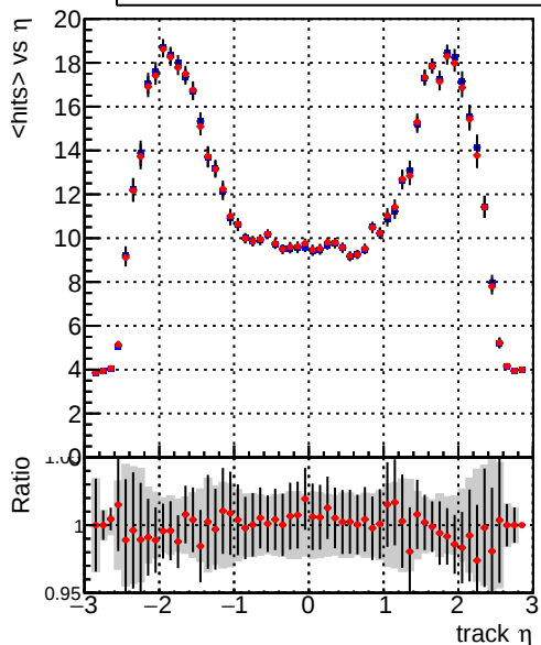
— DQM_mkFit_TT_baseline_6iter — DQM_mkFit_TT_RetrainV2_WP1_6iter mean hits
