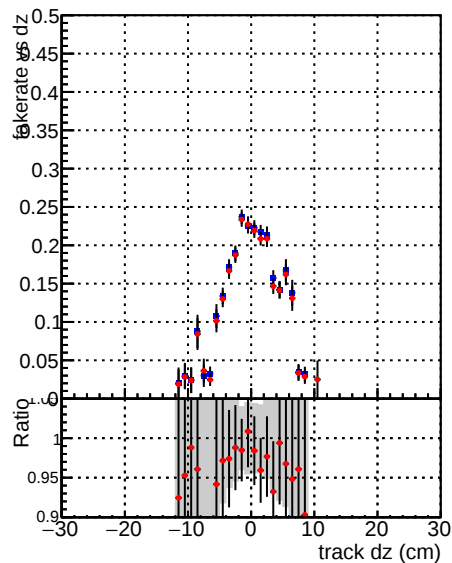
—●— DQM_mkFit_TT_baseline_6iter —●— DQM_mkFit_TT_RetrainV2_WP1_6iter
