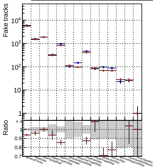
Number —●— DQM_mkFit_TT_RetrainV2_WP1_6iter
