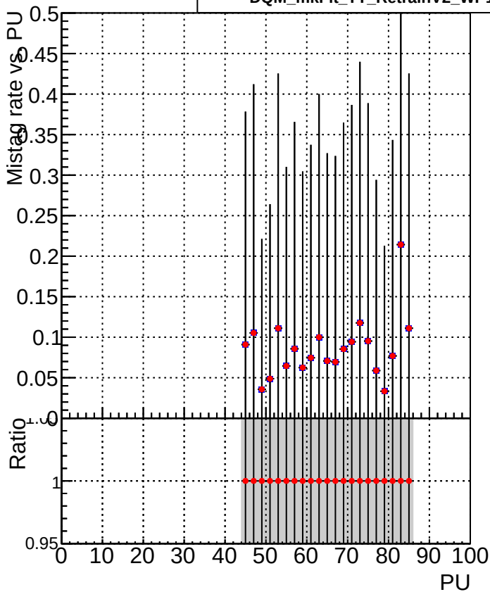
■ DQM_mkFit_TT_baseline_6iter ● DQM_mkFit_TT_RetrainV2_WP1_6iter
