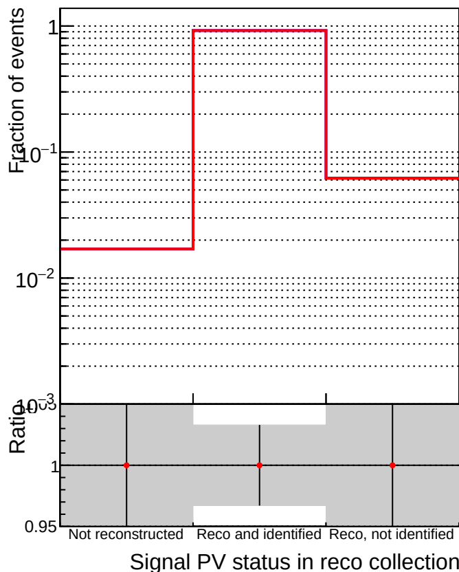
■ DQM_mkFit_TT_baseline_6iter ● DQM_mkFit_TT_RetrainV2_WP1_6iter
