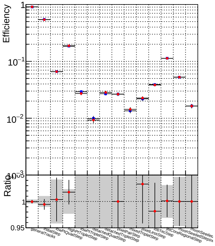
DQM_mkFit_TT_baseline_6iter DQM_mkFit_TT_RetrainV2_WP1_6iter
