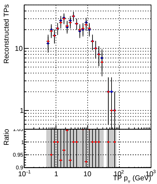
—●— DQM_mkFit_TT_baseline_6iter —◆— DQM_mkFit_TT_RetrainV2_WP1_6iter
