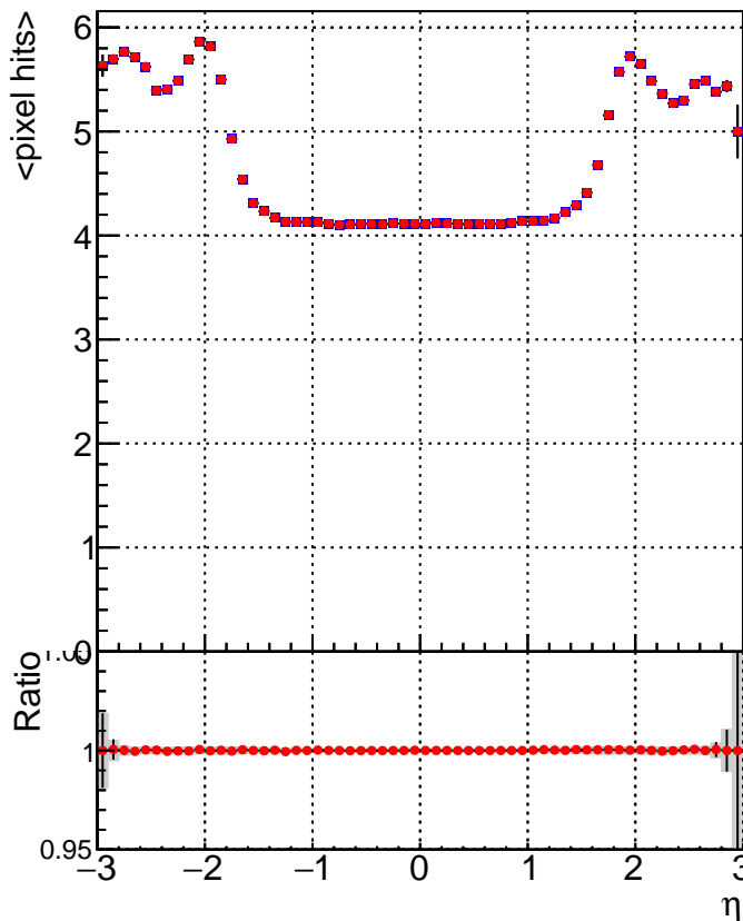
■ DQM_mkFit_TT_baseline_6iter ■ DQM_mkFit_TT_RetrainV2_WP1_6iter
