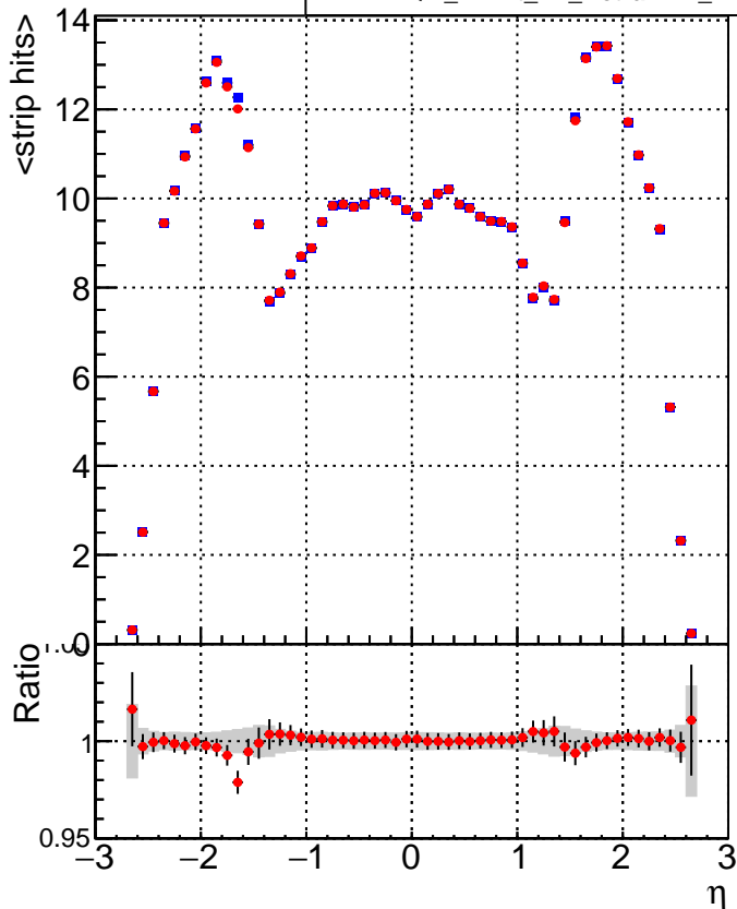
■ DQM_mkFit_TT_baseline_6iter ■ DQM_mkFit_TT_RetrainV2_WP1_6iter
