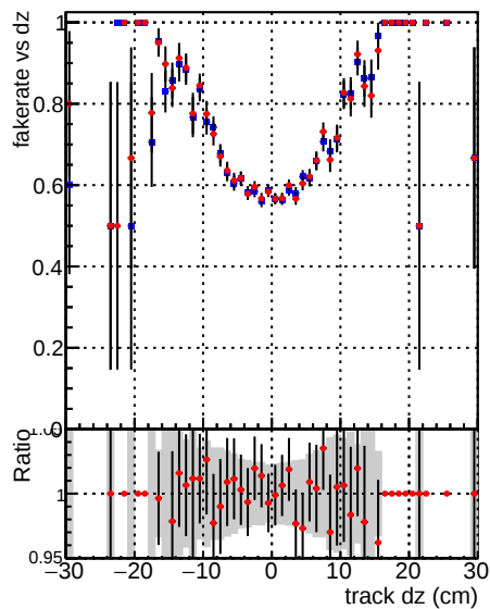
—●— DQM_mkFit_TT_baseline_6iter —●— DQM_mkFit_TT_RetrainV2_WP1_6iter
