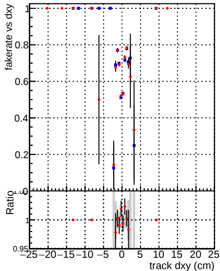
—●— DQM_mkFit_TT_baseline_6iter —●— DQM_mkFit_TT_RetrainV2_WP1_6iter
