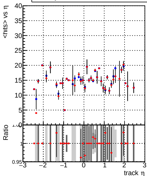
— DQM_mkFit_TT_baseline_6iter — DQM_mkFit_TT_RetrainV2_WP1_6iter
